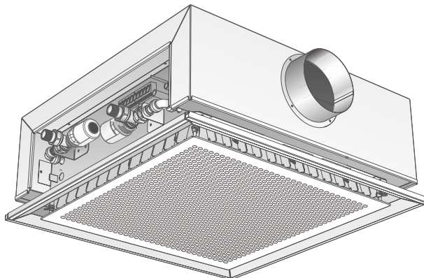
Figura 12. Sistema de regulación LUNA montado de fábrica. (Parasol T-RK-LUNA)
