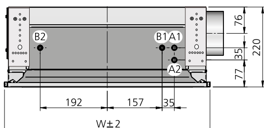
Figura 25. Parasol 600, vista lateral y conexiones A1 = Alimentación del agua de refrigeración \varnothing 12 \times 1,0 mm (Cu) A2 = Retorno del agua de refrigeración \varnothing 12 \times 1,0 mm (Cu) B1 = Alimentación del agua de calefacción \varnothing 12 \times 1,0 mm (Cu) B2 = Retorno del agua de calefacción \varnothing 12 \times 1,0 mm (Cu)
