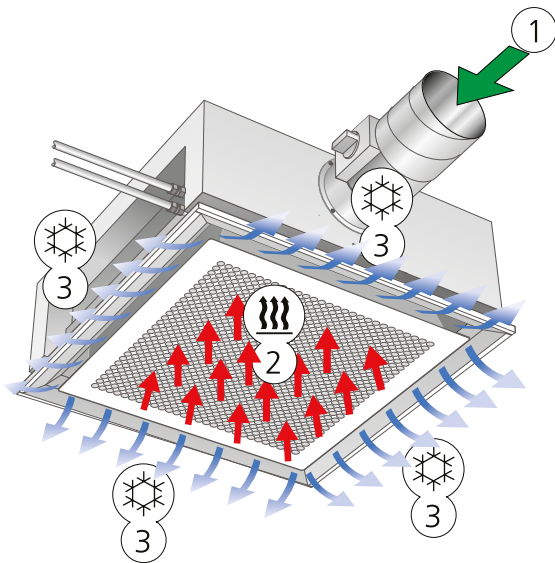
Figura 1. Versión A: Refrigeración y ventilación
