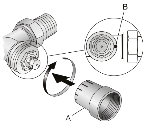
Figura 16. Ajuste del valor k_v A = Protector, se puede girar hasta 180° B = Marca en el lado de salida de la válvula
