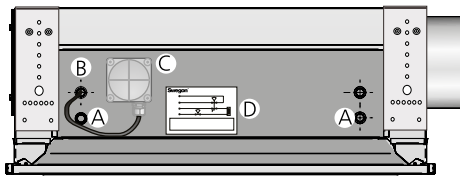
Figura 29. Parasol 1200 para calefacción eléctrica, visto desde el lateral de conexiones
