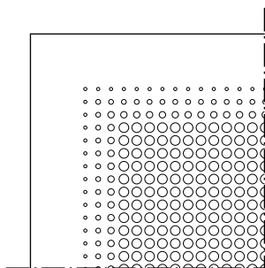
Figura 10. Chapa frontal PD Orificios circulares dispuestos en un diseño cuadrado con el borde en disminución.
