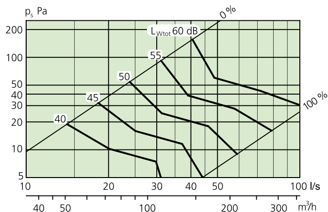
Gráfico 7. Rango de ajuste, compuerta CRPc 9-125
