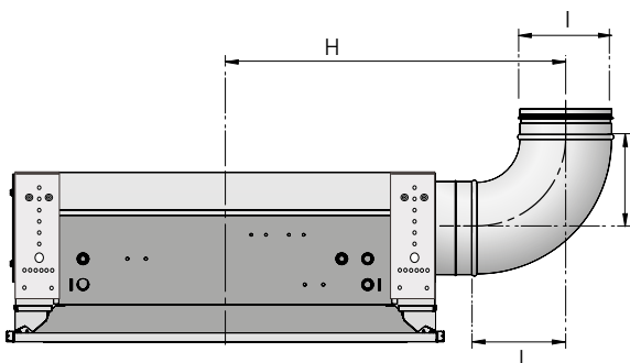
Figura 31. Conexión con codo, vista lateral Pieza de conexión montada SYST CA xxx-90
