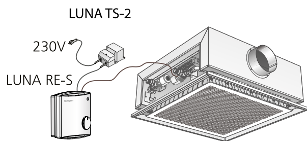
Figura 14. Instalación típica, refrigeración y calefacción por agua
