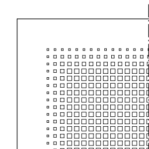
Figura 11. Chapa frontal PE Orificios cuadrados dispuestos en un diseño cuadrado con el borde en disminución.
