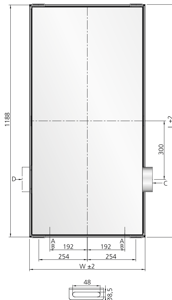
Figura 28. Parasol 1200, vista superior A = Alimentación y retorno del agua de refrigeración \varnothing 12 \times 1,0 mm (Cu) B = Alimentación y retorno del agua de calefacción \varnothing 12 \times 1,0 mm (Cu) C = Pieza de conexión para aire primario \varnothing 125 mm (PF = \varnothing 160 mm) D = Conexión de aire alternativa tapada
