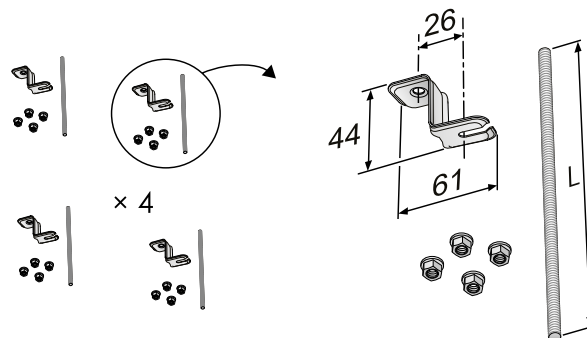
Figura 20. Conjunto de montaje SYST MS-1, fijación para techo y varilla roscada.
