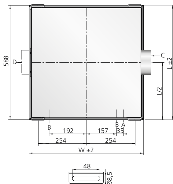
Figura 26. Parasol 600, vista superior A = Alimentación y retorno del agua de refrigeración \varnothing 12 \times 1,0 mm (Cu) B = Alimentación y retorno del agua de calefacción \varnothing 12 \times 1,0 mm (Cu) C = Pieza de conexión para aire primario \varnothing 125 mm D = conexión de aire alternativa tapada
