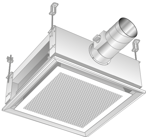
Figura 17. Fijación al techo de una unidad sencilla
