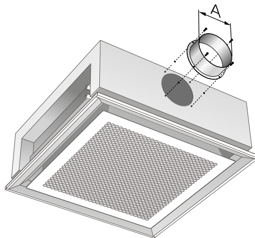
Figura 19. Pieza de conexión del aire
