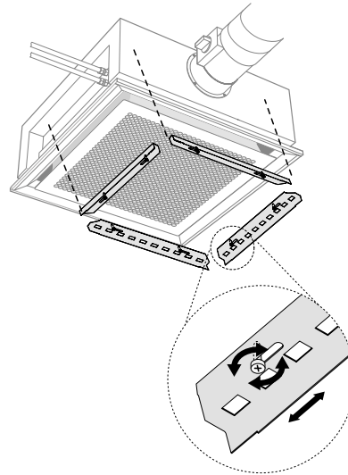
Figura 5. Ajuste de las boquillas
