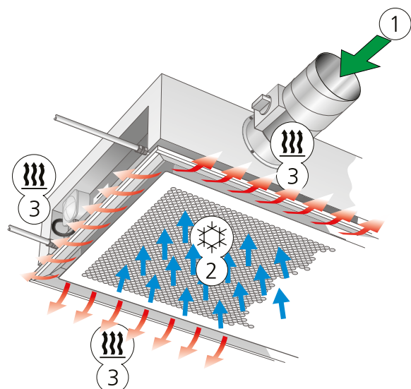
Figura 4. Versión X: Ventilación y calefacción con elementos calefactores eléctricos (incluye también modo de refrigeración)
