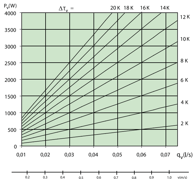
Gráfico 5. Caudal de agua – Potencia calorífica
