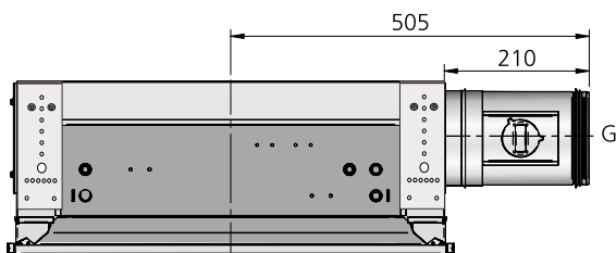
Figura 30. Conexión con compuerta, vista lateral Compuerta de ajuste montada SYST CRPc 9-xxx
