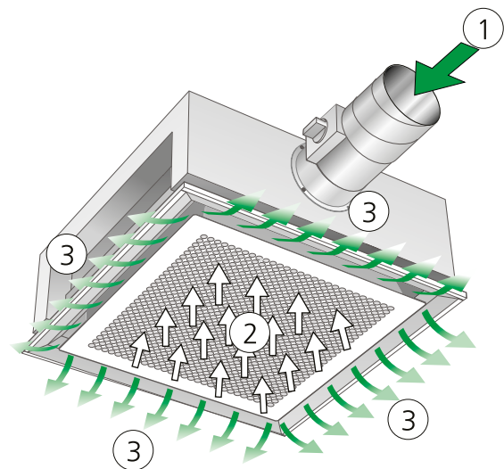
Figura 3. Versión C: Ventilación
