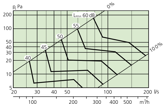
Gráfico 8. Rango de ajuste, compuerta CRPc 9-160
