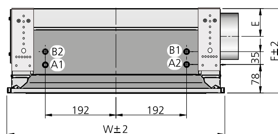
Figura 27. Parasol 1200, vista lateral y conexiones A1 = Alimentación del agua de refrigeración \varnothing 12 \times 1,0 mm (Cu) A2 = Retorno del agua de refrigeración \varnothing 12 \times 1,0 mm (Cu) B1 = Alimentación del agua de calefacción \varnothing 12 \times 1,0 mm (Cu) B2 = Retorno del agua de calefacción \varnothing 12 \times 1,0 mm (Cu)
