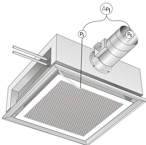
Figura 24. Condiciones de presión - Aire
