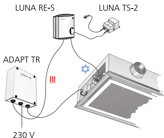
Figura 15. Instalación, refrigeración por agua y calefacción eléctrica
