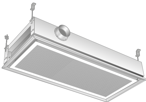
Figura 18. Fijación al techo de una unidad doble
