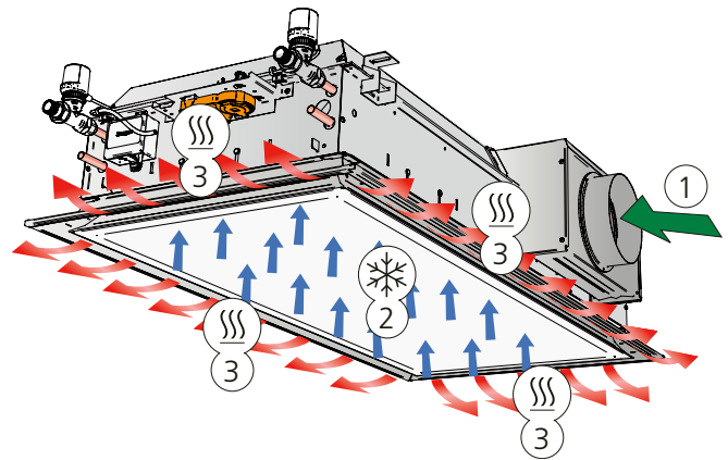
Figure 4. Variante B : Chauffage et ventilation (inclut également une fonction de refroidissement)
