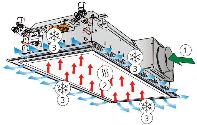
Figure 3. Variante A : Refroidissement et ventilation
