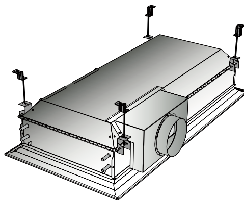
Figure 22. Unités à double module en suspension
