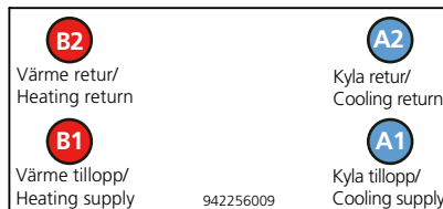
Figure 28. Raccord hydraulique – Longueur 600, 1200 et 1800* A1 = Alimentation eau glacée Ø12 x 1,0 mm (Cu) A1 = Alimentation eau glacée Ø15 x 1,0 mm (Cu) *(Taille 1800) A2 = Retour eau glacée Ø12 x 1,0 mm (Cu) A2 = Retour eau glacée Ø15 x 1,0 mm (Cu) *(Taille 1800) B1 = Alimentation eau chaude Ø12 x 1,0 mm (Cu) B2 = Retour eau chaude Ø12 x 1,0 mm (Cu)
