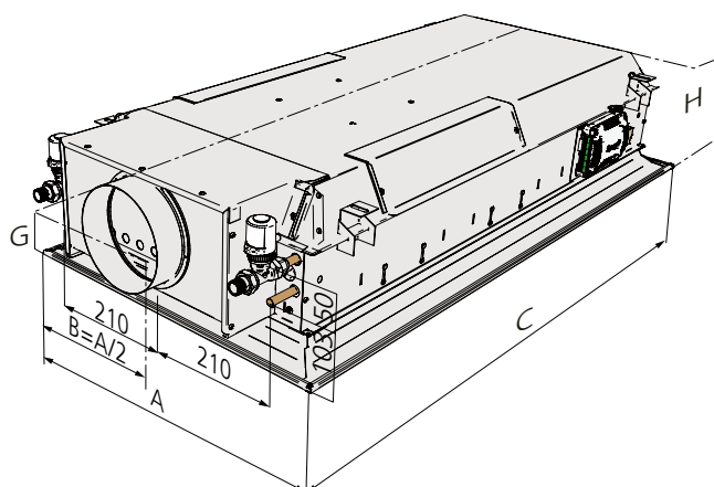
Figure 31. Schéma de dimensionnement – raccordement sur côté court (l'exemple montre une longueur 1200 avec raccordement aéraulique sur le côté 1).
