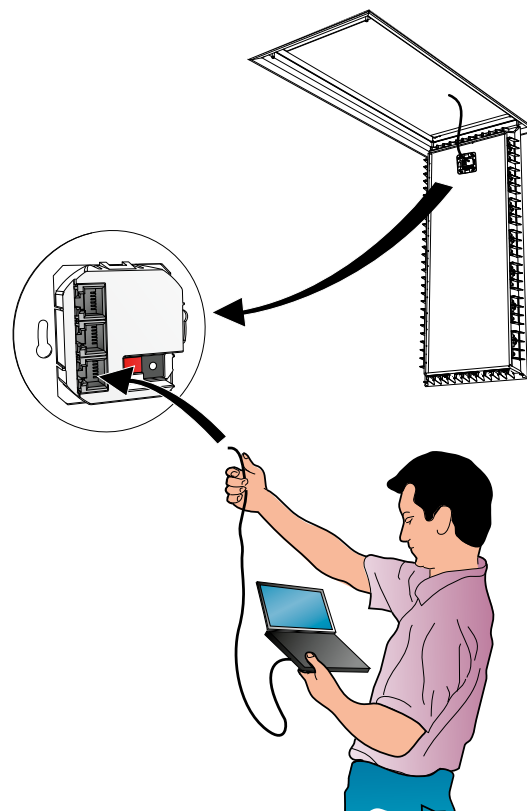
Figure 10. Le CÂBLE CONVERTISSEUR USB-RJ12 (RS485) permet de raccorder un PC au système (pour configurer le logiciel, par exemple). Le câble se branche soit à l'arrière du module de détection (comme illustré), ou directement sur le régulateur. Pour le détail de la procédure, voir le mode d'emploi SWICCT.
