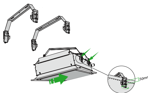
Figure 24. Fixation au moyen du KIT DE SUSPENSION RAPIDE PARASOL Z
