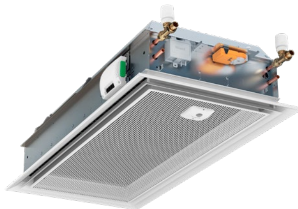
Figure 1. PARASOL Zenith AWC avec composants installés en usine : régulateur, vannes, servomoteurs et module de détection.
