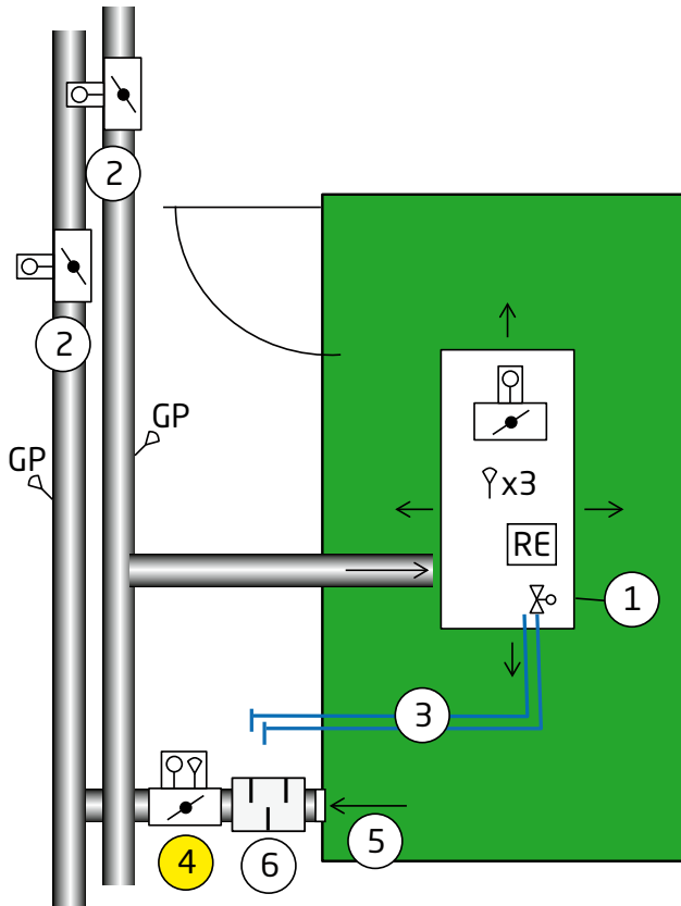
Figure 11. Le local type montre un PARASOL Zenith AWC installé dans un bureau
