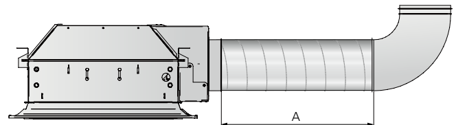
Figure 29. Schéma de dimensionnement, raccordement côté longueur, avec coude Ø125/160/200
