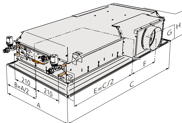
Figure 30. Schéma de dimensionnement – raccordement sur côté long (l'exemple montre une longueur 1200 avec raccordement aéraulique sur le côté 2).
