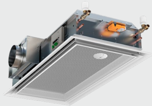
WISE Parasol Zenith med ställdon, vattenanslutning, ventilställdon på sida 1 samt luftanslutning och WISE CU på sida 4
