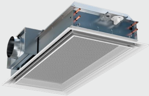
PARASOL Zenith med inställningsvred och vattenanslutning på sida 1 samt luftanslutning på sida 4
