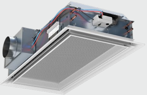
REACT Parasol Zenith med ställdon och vattenanslutning på sida 1 samt luftanslutning med flödesmätning på sida 4
