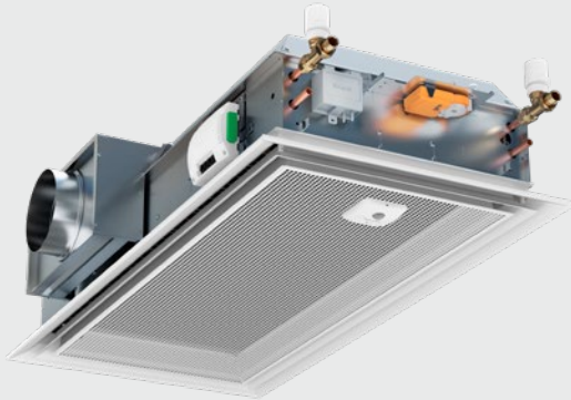
PARASOL Zenith AWC med ställdon, vattenanslutning, ventilställdon på sida 1 och luftanslutning och regulator på sida 4
