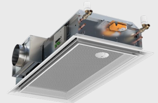
WISE PARASOL Zenith met aandrijving, wateraansluiting en klepactuator op zijde 1 en luchtaansluiting en WISE CU op zijde 4
