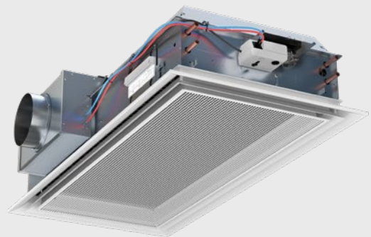
REACT Parasol Zenith met actuatoren en wateraansluiting op zijde 1 en luchtaansluiting met debietmeting op zijde 4
