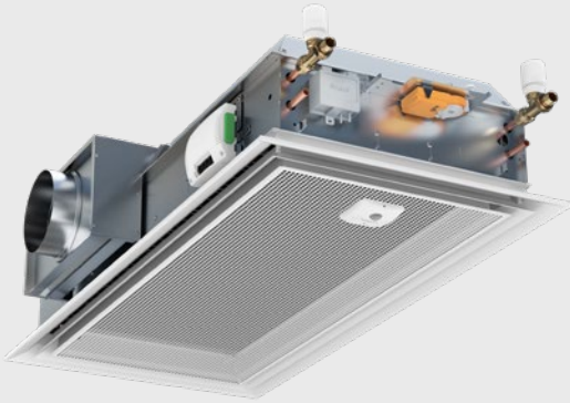
PARASOL Zenith AWC, jossa pellin toimilaite, vesiliitäntä ja venttiilitoimilaite sivulla 1 sekä ilmaliitäntä ja säädin sivulla 4
