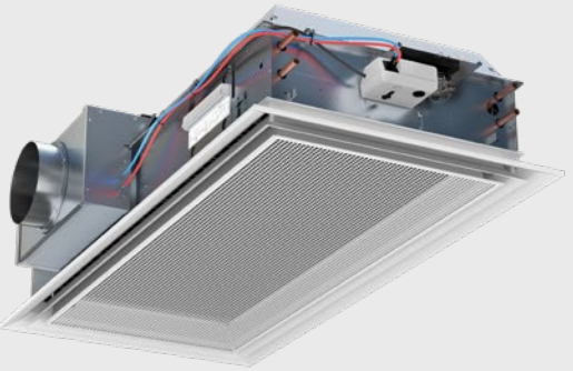
REACT Parasol Zenith toimilaitteilla ja vesiliitännällä sivulla 1 sekä ilmaliitännällä ja virtausmittauksella sivulla 4
