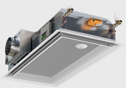
WISE PARASOL Zenith, jossa pellin toimilaite, vesiliitäntä ja venttiilitoimilaite sivulla 1 sekä ilmaliitäntä ja WISE CU sivulla 4
