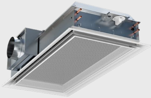
PARASOL Zenith, jossa säätönuppi ja vesiliitäntä sivulla 1 ja ilmaliitäntä sivulla 4
