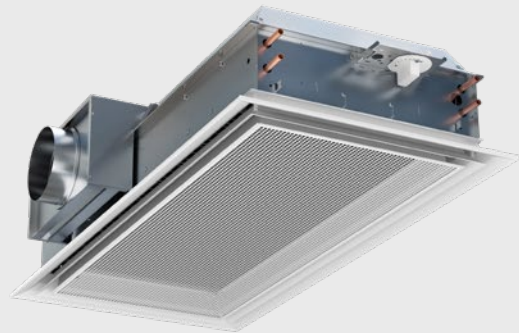
PARASOL Zenith, med indstillingsgreb og vandtilslutning på side 1 og lufttilslutning på side 4
