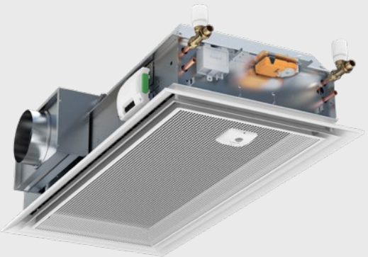
PARASOL Zenith AWC, med aktuator, vandtilslutning, ventilmotor på side 1 og lufttilslutning og regulator på side 4
