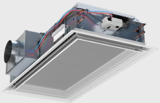
REACT Parasol Zenith med aktuator og vandtilslutning på side 1 samt lufttilslutning med luftmængdemåling på side 4
