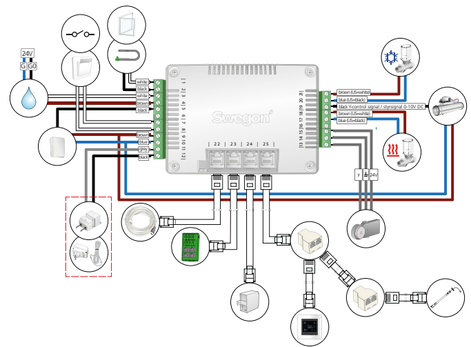
Abb. 5. Regler URC1.
