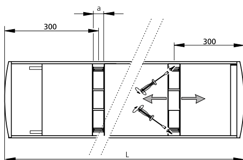
Figura 10. Connessione -I, vista dall'alto.
