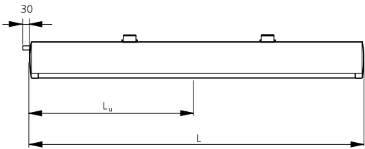
Figura 7. Connessione -H, vista laterale. A = lunghezza FRB L_u = Misura verso la suddivisione della parte inferiore
