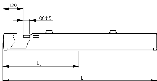
Figura 9. Connessione -I, vista laterale.
