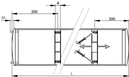
Figura 8. Connessione orizzontale nel lato corto -H, vista dall'alto. a = spazio di regolazione per l'attacco 43 mm.
