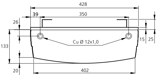
Figura 6. FRB, vista dal lato corto.
