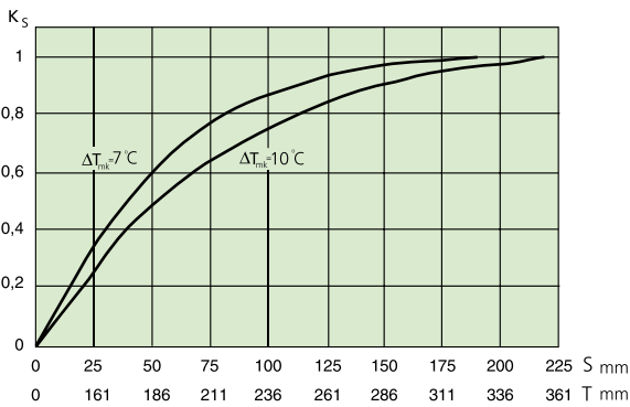
Diagramma 4. spazio per la circolazione dell'aria
