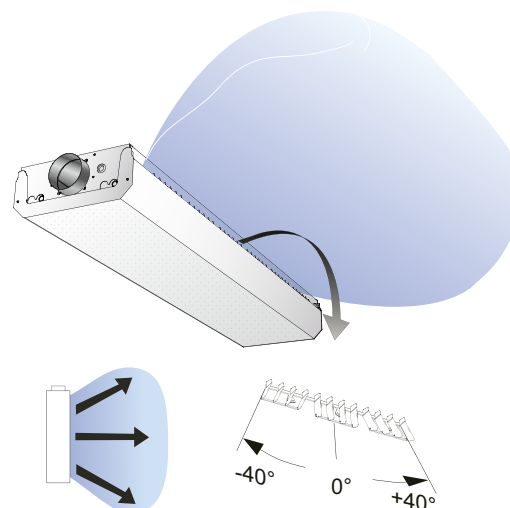
Figure 6. Options de réglage de l'ADC, en éventail
