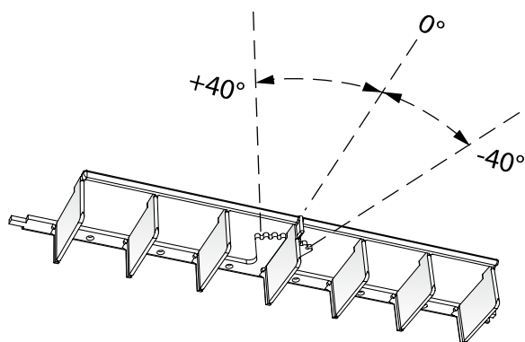
Figure 5. Déflecteurs d'air Swegon ADC.
