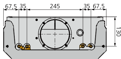
Figure 15. Dimensions ADRIATIC Prisma, vue arrière du raccordement hydraulique
