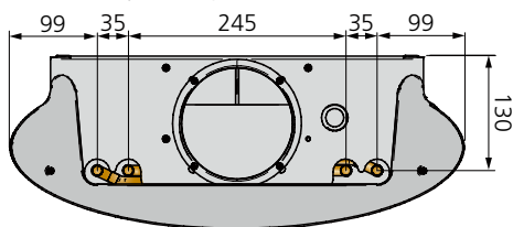
Figure 16. Dimensions ADRIATIC Ellips, vue arrière du raccordement hydraulique
