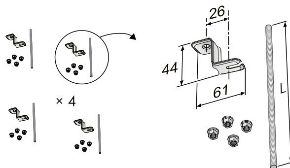
Figure 10. Accessoire d'installation SYST MS M8-1, montage au plafond et sur tige filetée
