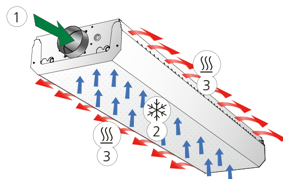
Figure 4. Chauffage et ventilation
