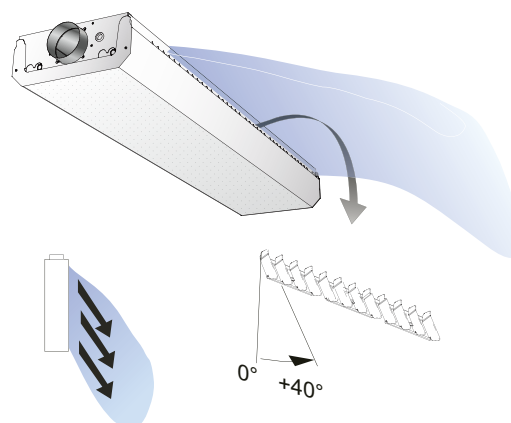
Figure 7. Options de réglage de l'ADC, en X
