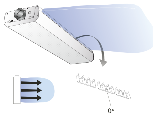
Figure 8. Options de réglages ADC, diffusion perpendiculaire
