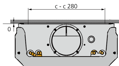
Figure 23. Installation – montage suspendu à l'aide de l'accessoire SYST MS-M8.
