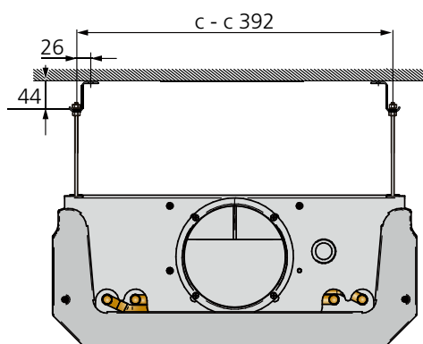
Figure 23. Installation – montage suspendu à l'aide de l'accessoire SYST MS-M8.
