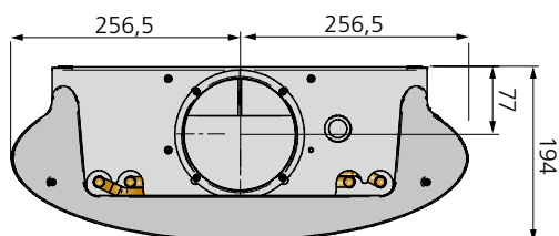
Figure 20. Dimensions ADRIATIC Ellips, vue arrière du raccordement aéraulique
