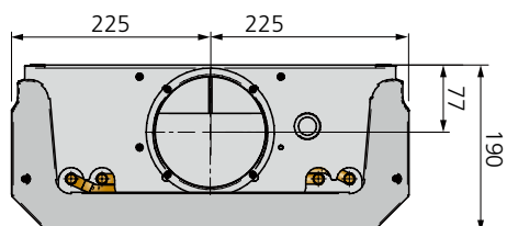
Figure 19. Dimensions ADRIATIC Prisma, vue arrière du raccordement aéraulique
