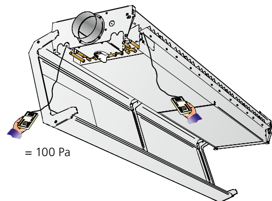
Figure 14. Les tubes de mesure se situent sur les deux longs côtés du produit.
