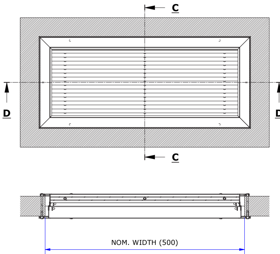
SECTION D-D
