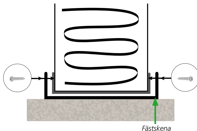
Figur 1. Montera fästskena
