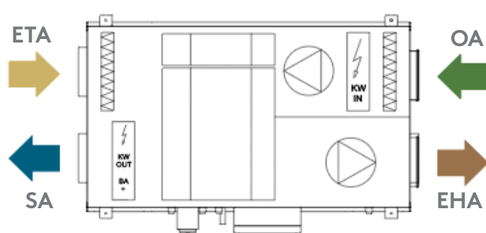
GLOBAL PX LP (WIDOK Z GÓRY)
