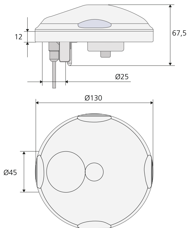
Figuur 2. Afmetingen, WISE WS.
