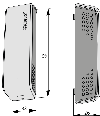
Figur 2. Mått, WISE WCS
