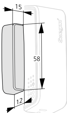
Figur 3. Mått, WISE WCS magnet.
