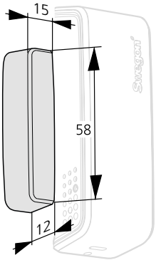
Figure 3. Dimensions, module magnétique WISE WCS
