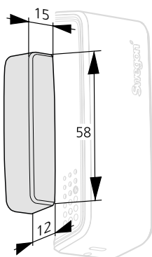
Kuva 3. Mitat, WISE WCS magneetti.
