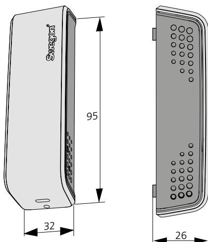
Kuva 2. Mitat, WISE WCS
