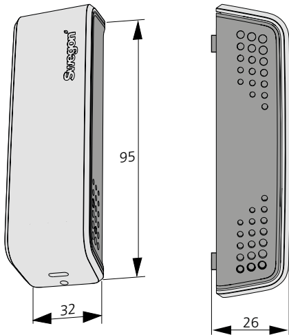
Abb. 2. Abmessungen, WISE WCS
