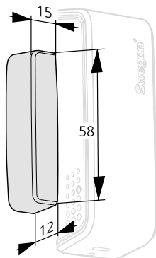
Abb. 3. Abmessungen, WISE WCS-Magnet.
