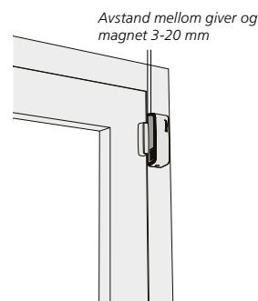
Figur 1. Anbefalt plassering av WISE WCS.
