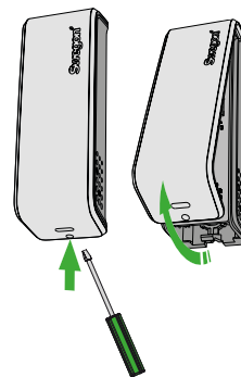
Figur 3a. Ta av forstykket. Demonter alltid produktet i denne retningen.
