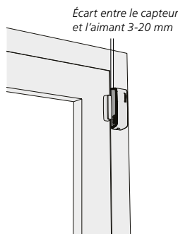
Figure 1. Emplacement recommandé de la sonde WISE WCS.
