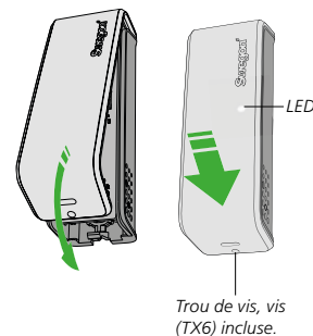
Figure 3b. Fixer la partie avant. Procéder toujours dans ce sens pour installer le produit.
