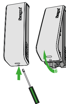
Figure 3a. Retirer la partie avant. Procéder toujours dans ce sens pour démonter le produit.
