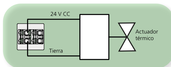
Conexión del actuador térmico
