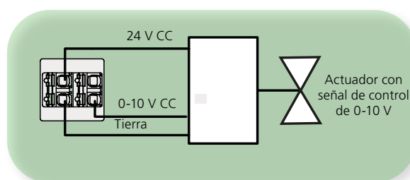
Conexión del actuador con señal de control de 0-10 V. NOTA Alimentación 24 V CC
