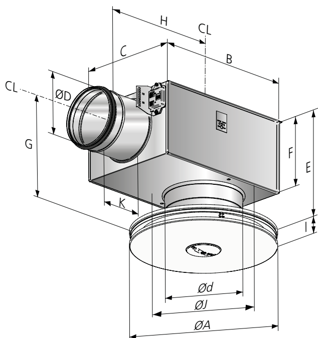
Figura 1. WISE Sphere C, esquema de dimensiones.
