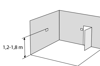
Figur 1. Anbefalt plassering av WISE RTS.
