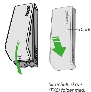
Figur 3b. Sett på forstykket. Monter alltid produktet i denne retningen.
