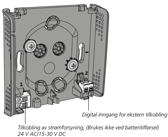
Figur 4. Bakstykke. Bakstykket kan monteres på vegg, eventuelt i apparatkabinett. Bakstykket er klargjort med knockouts for kabelgjennomføring.
