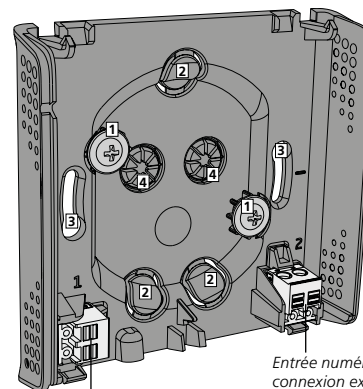
Raccordement de l'alimentation 24 V CA/15-30 V CC (Pas utilisé pour l'alimentation par batterie)
