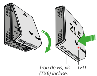
Figure 3b. Fixer la partie avant. Procéder toujours dans ce sens pour installer le produit.
