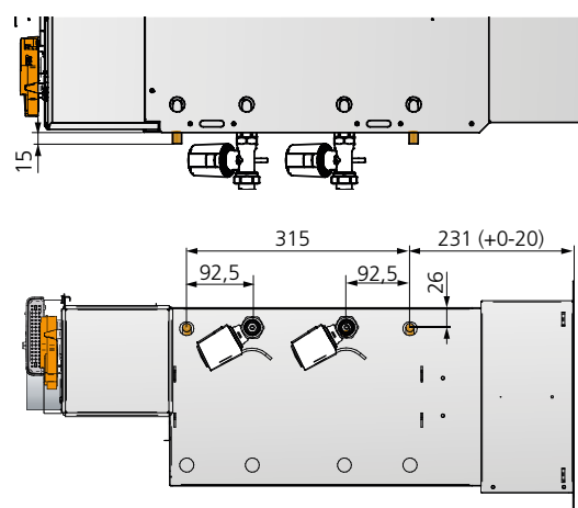
Figura 18. Dimensioni del raccordo per l'acqua
