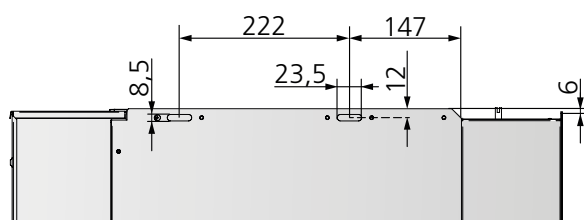
Figura 14. Dimensioni della sospensione
