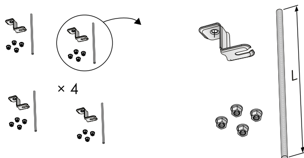
Figura 15. Raccordo di montaggio SYST MS M8-1, supporto per soffitto e asta filettata
