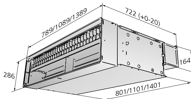
Figura 20. Schema delle quote senza griglia
