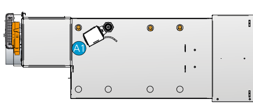
Figura 17. Raccordo per l'acqua sul lato destro (R).
