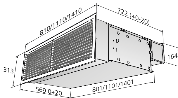
Figura 21. Schema delle quote con griglia
