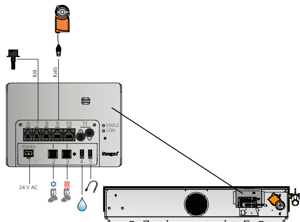
Figur 2. Komponenterna som kan fabriksmonteras på WISE Paragon
