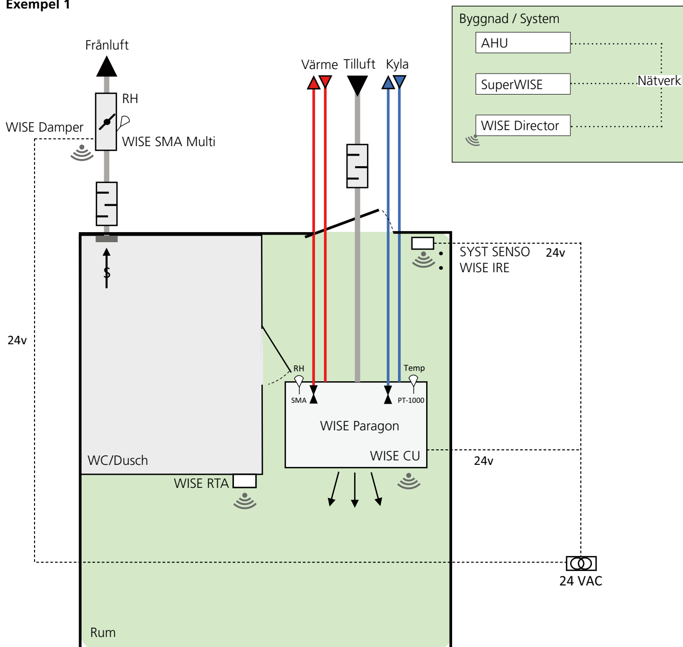
Figur 14. Hotellösning med WISE Paragon, exempel 1
