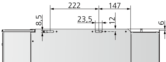
Figur 16. Mått upphängning
