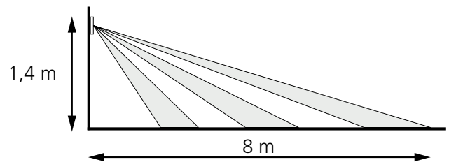
Kuva 2. Tunnistusalue, seinäasennus.
