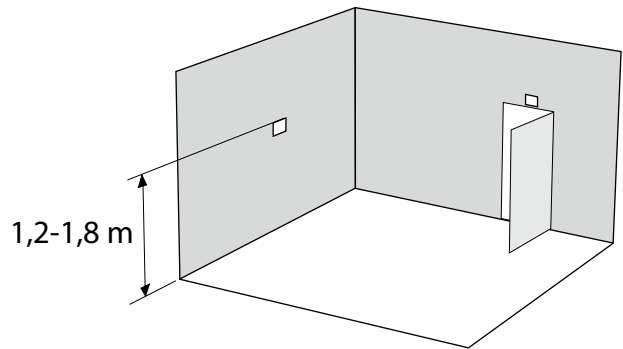
Kuva 1. WISE OCS:n asennus seinälle.
