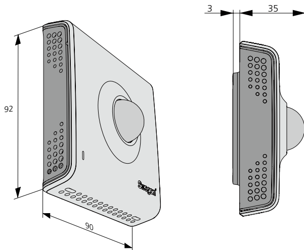
Kuva 4. Mitat, WISE OCS.
