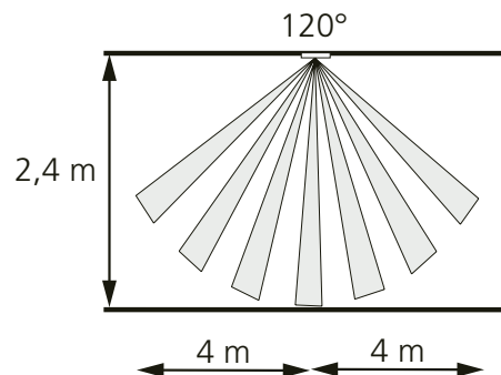
Kuva 3. Tunnistusalue, kattoasennus.
