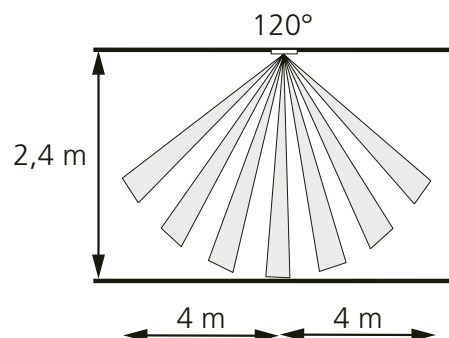
Abb. 3. Erfassungsbereich, Deckenmontage.
