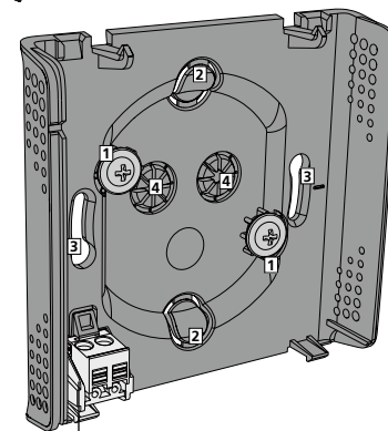
Raccordement de l'alimentation 24 V CA/15-30 V C
