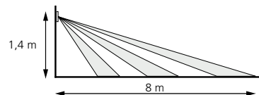
Figure 1. Champ de détection, montage mural.
