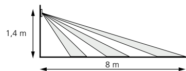
Abb. 1. Erfassungsbereich, Wandmontage.
