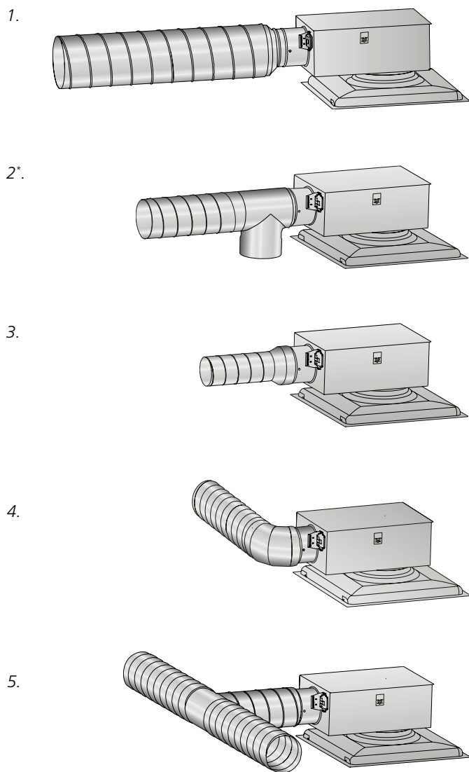
Figur 3. Krav raksträcka cirkulära kanaler.
