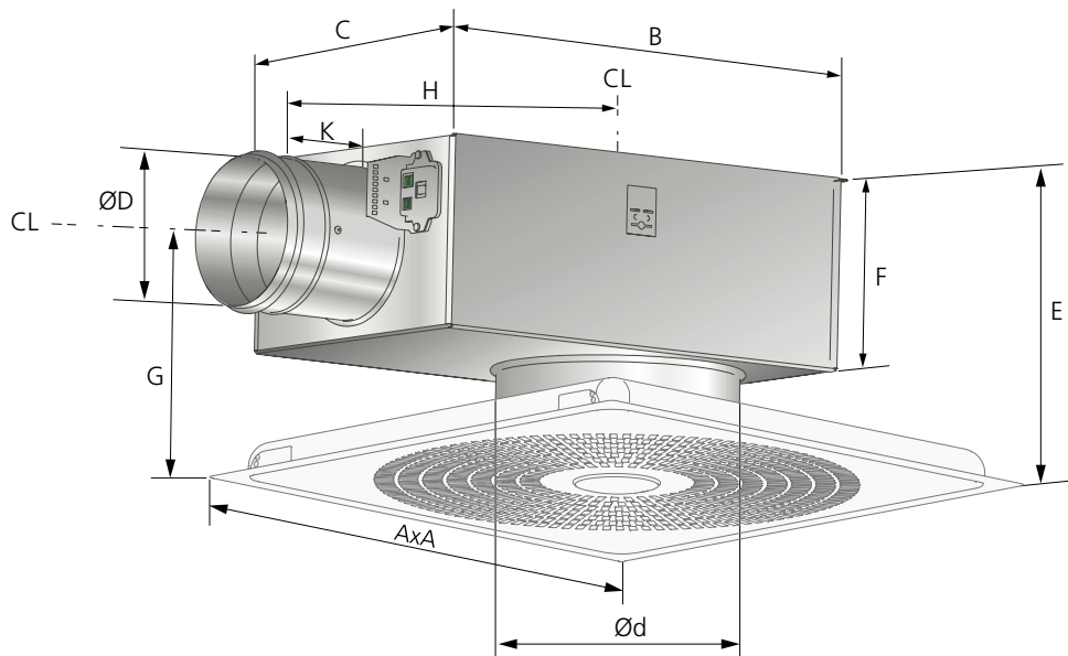
Figur 2. WISE Lockzone Ceiling, måttfigur.
