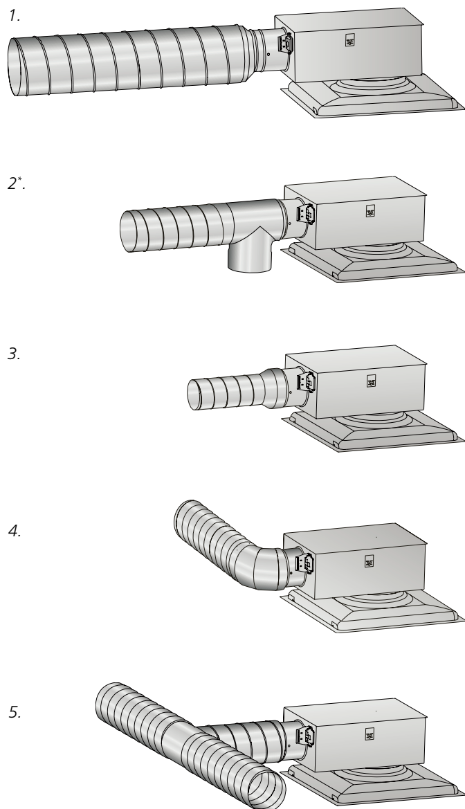
Figur 4. Krav til rettstrekning i sirkulære kanaler.
