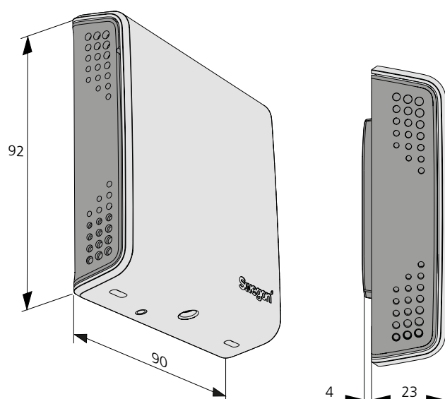
Figur 3. Mått, WISE IRT.
