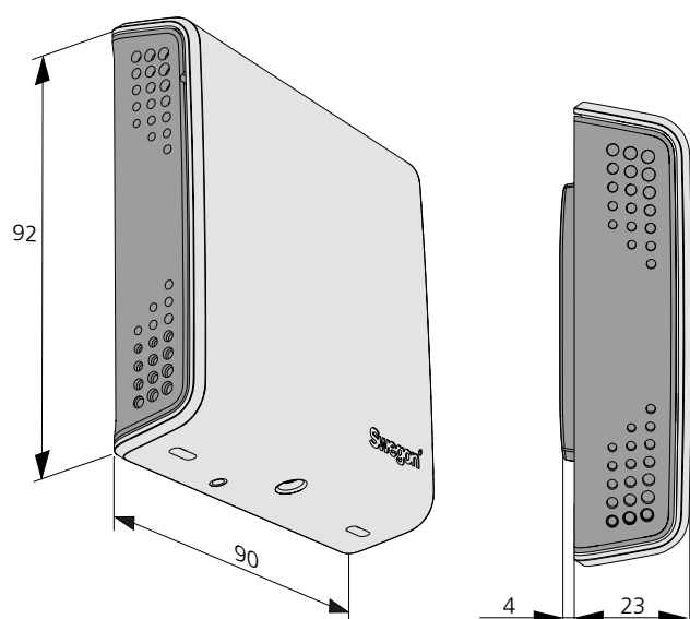
Figur 3. Mål, WISE IRT.
