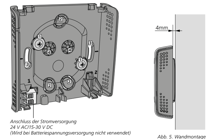
Abb. 4. Rückteil.
