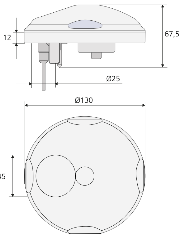
Figur 4. Mått, WISE WS.
