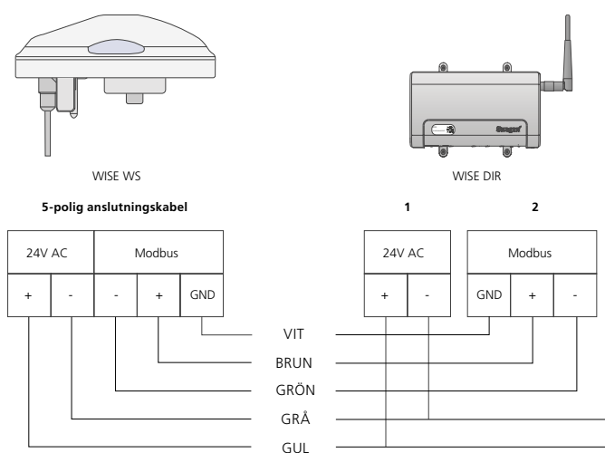
5-polig anslutningskabel
