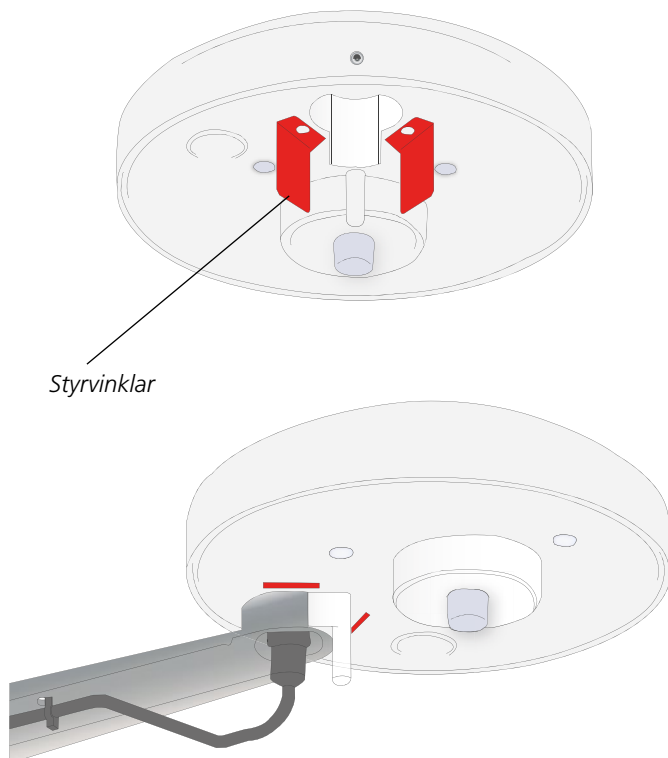
Figur 1. Montering med väggfäste.
