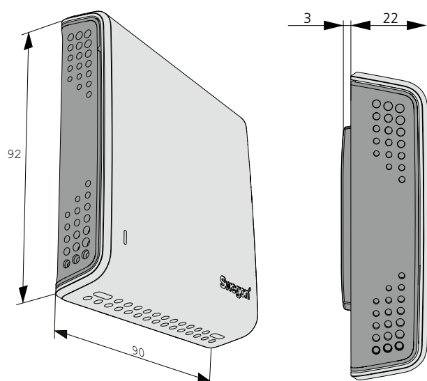
Figur 3. Mått, WISE IAQ.
