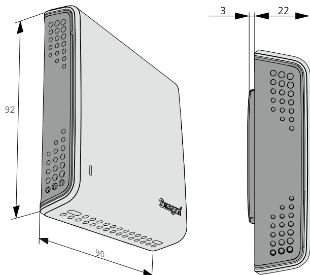
Kuva 3. Mitat, WISE IAQ.
