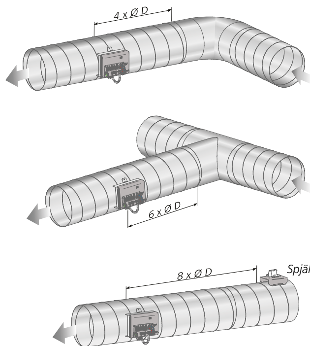
Figur 4. Krav på raksträckor före WISE DPS.
