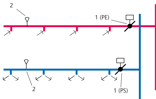
Figur 2. Konstantrykkregulering, anbefalt installasjon 2/3 ut i kanalen.
