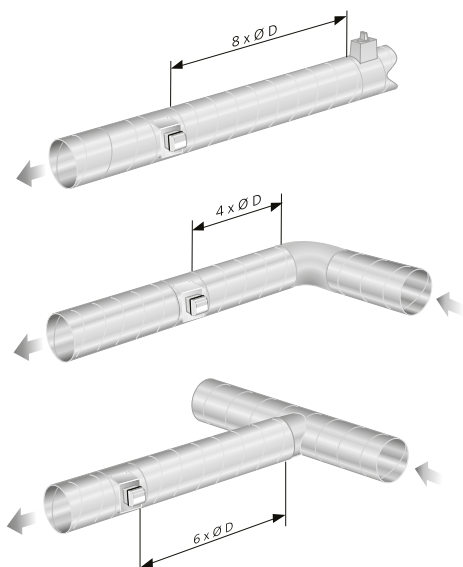
Kuva 3. Vaatimus suorasta osuudesta ennen WISE DPS Modbusia.
