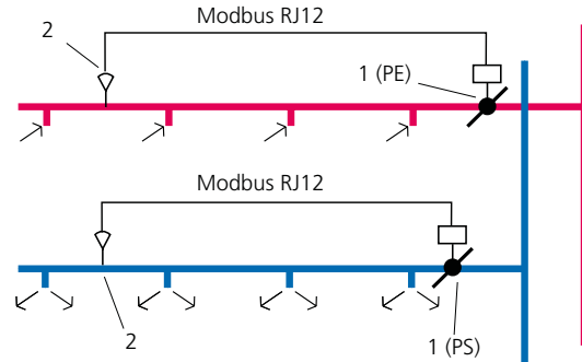
Kuva 1. Vakiopainesäätö, suositeltu asennus 2/3 kanavaan, maks. 100 m.
