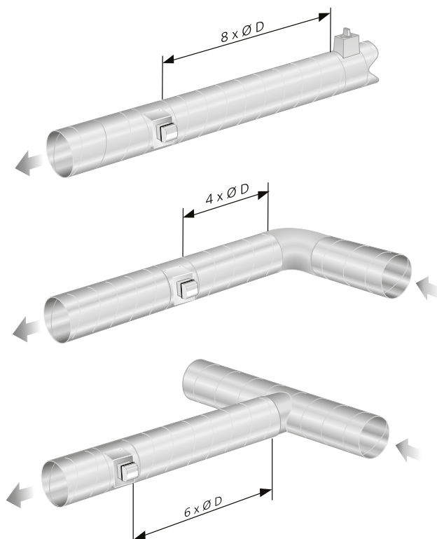
Figur 4. Krav på raksträckor före WISE DPS Modbus.
