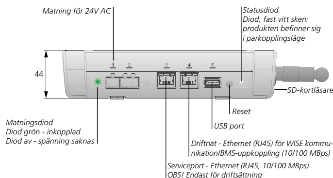
Figur 2. Kabelinkoppling och mått.
