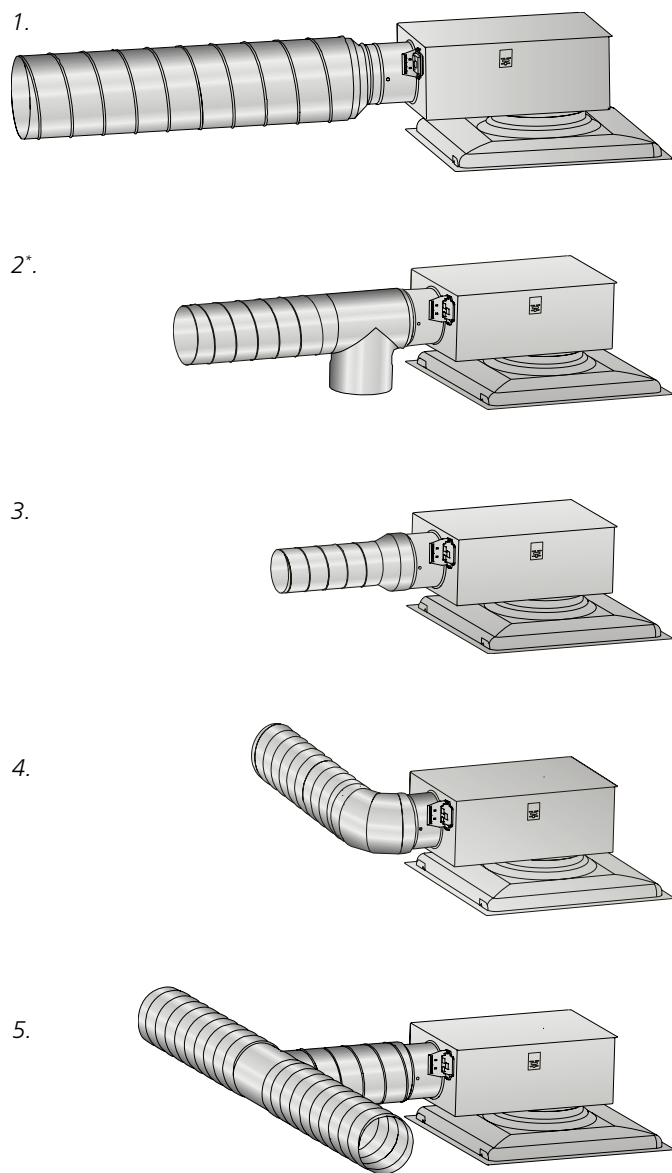
Figur 4. Krav på raksträcka i cirkulära kanaler.
