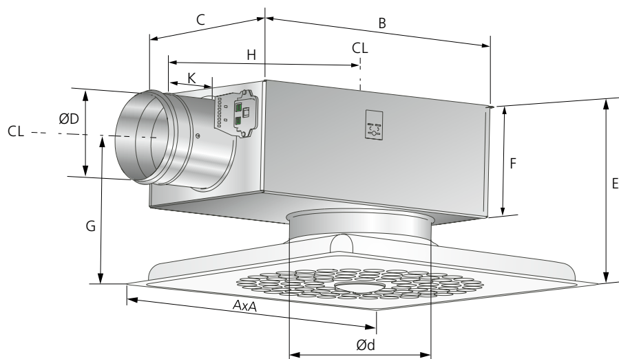
Figur 2. WISE Colibri Ceiling, måttfigur.
