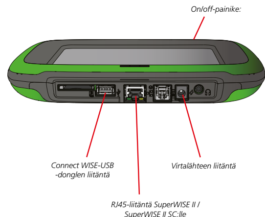
Kuva 2. TuneWISE -käsipäätteen liitännät.
