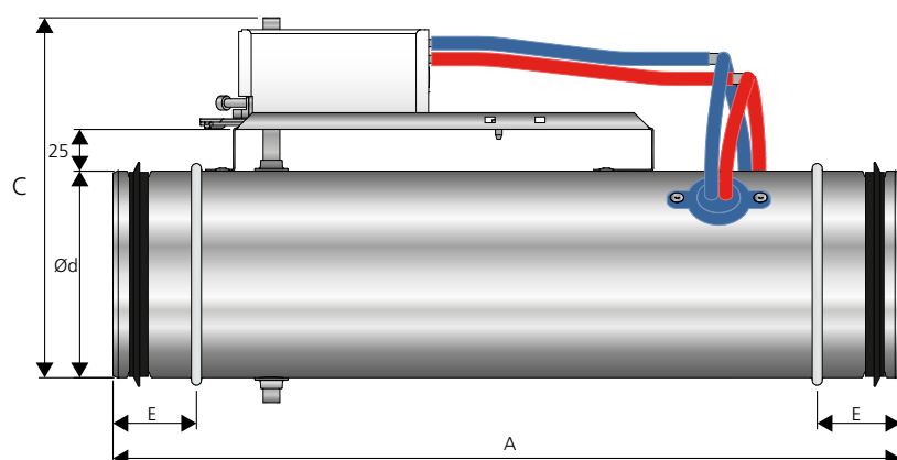
Figur 4. Mål (mm), REACT V SKNX sirkulær. Spjeld kan monteres i valgfri vinkel.
