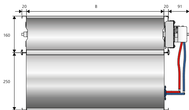
Figur 8. Mål (mm), REACT V SKNX rektangulær.
