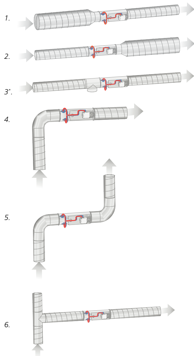
Figur 5. Krav til rettstrekning i sirkulære kanaler, antall \varnothing før produkt: Bilde 1–5 krever ingen rettstrekning (bilde 3* illustrerer T-stykke med renseluke). Bilde 6 krever rettstrekning før spjeldet tilsvarende 4 \times kanalens diameter.
