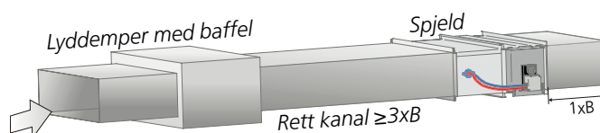
Figur 11. Krav til rettstrekning 3 \times B ved lyddemper med baffel. Gjelder både til- og fraluft.
