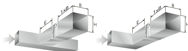
Figur 10. Krav til rettstrekning i rektangulære kanaler.
