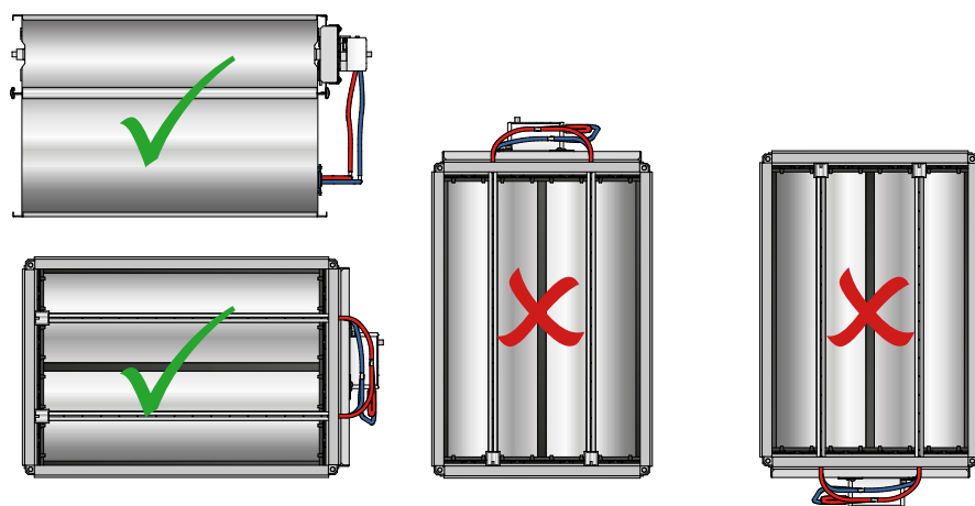
Figur 9. Montering -For rektangulære kanaler monteres alltid spjeldet slik at regulatoren/aktuatoren er plassert langs siden på kanalen.
