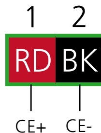
Figur 2. Kommunikasjon (grønn kabel).
