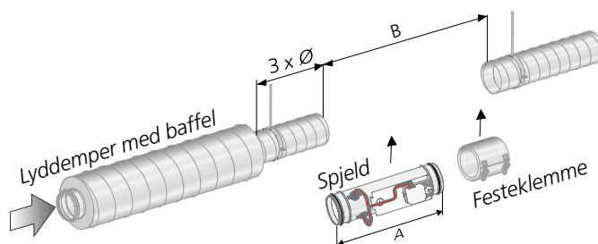
Figur 6. Krav til rettstrekning 3 \times \varnothing ved lyddemper med baffel eller akustisk kjerne.
