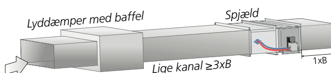
Figur 11. Krav til lige strækning 3 \times B ved lyddæmper med baffel. Gælder både til- og fraluft.
