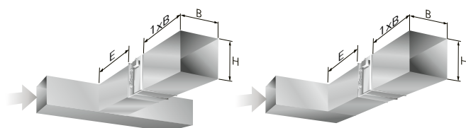
Figur 10. Krav til lige strækning i rektangulære kanaler.
