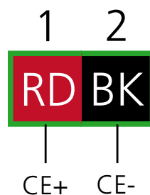
Figur 2. Kommunikation (grønt kabel).
