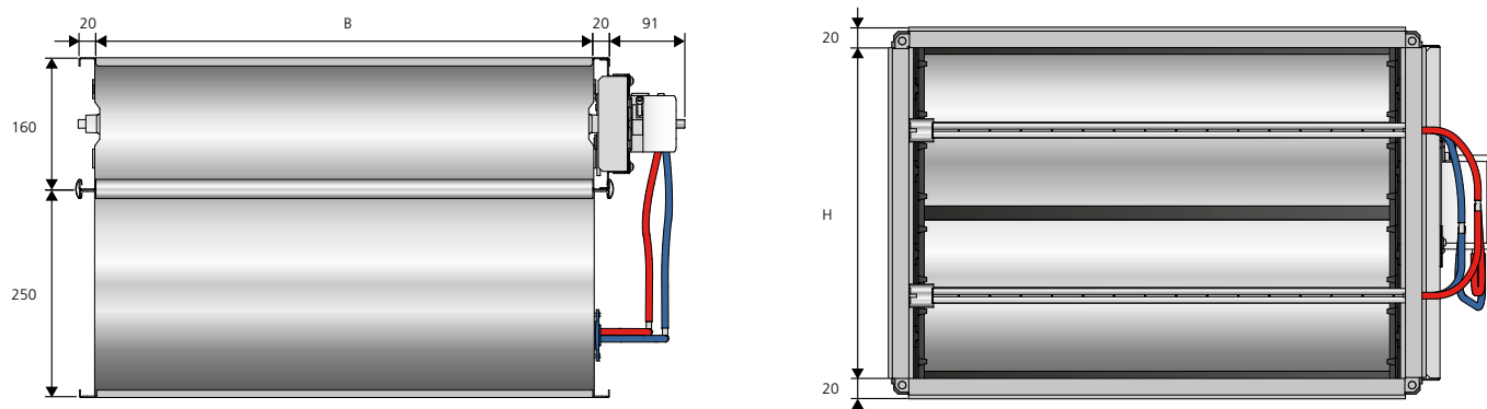
Figur 8. Mål (mm), REACT V SKNX rektangulær.
