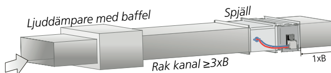
Figur 10. Krav på raksträcka 3 \times B vid ljuddämpare med baffel. Gäller både till- och frånluft.
