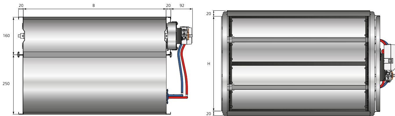
Figur 7. Mått (mm), REACT V GMB rektangulär.
