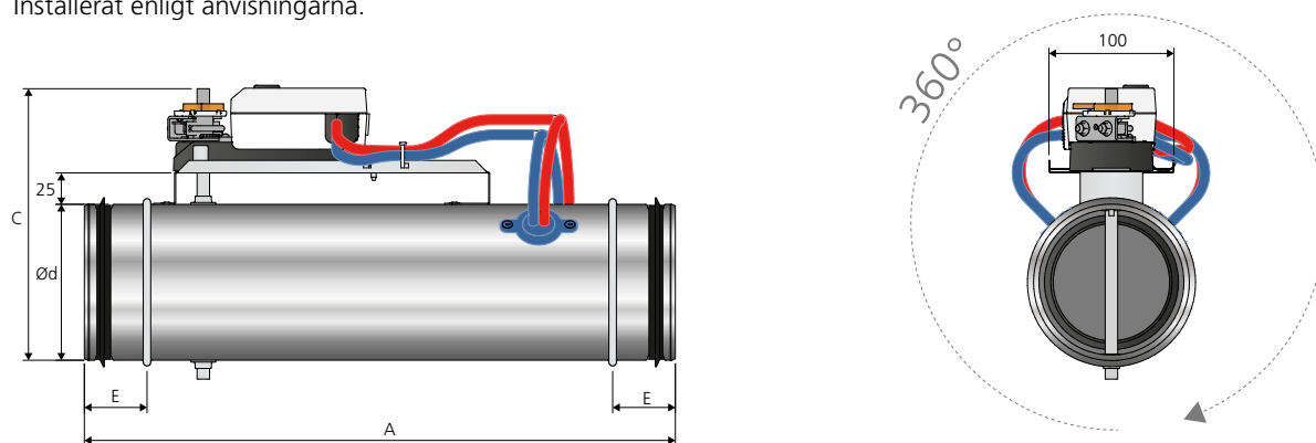
Figur 3. Mått (mm), REACT V GMB cirkulär. Spjäll kan monteras i valfri vinkel.
