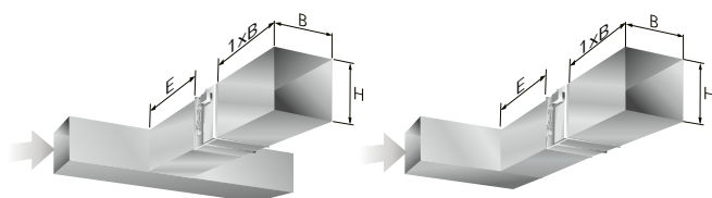
Figur 9. Krav til lige strækning i rektangulære kanaler.
