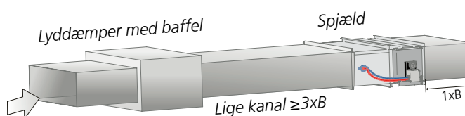
Figur 10. Krav til lige strækning 3 \times B ved lyddæmper med baffel. Gælder for både tilluft og fraluft.
