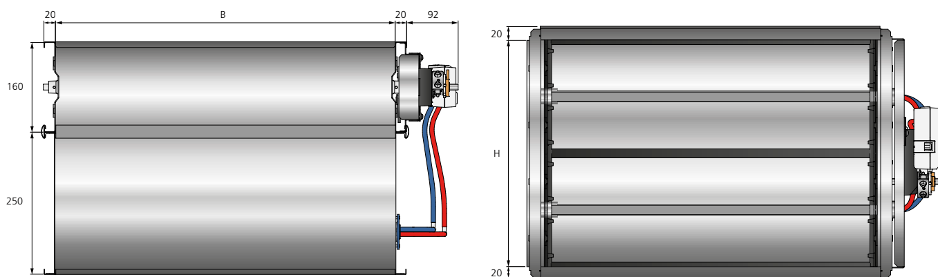
Figur 7. Mål (mm), REACT V GMB rektangulær.
