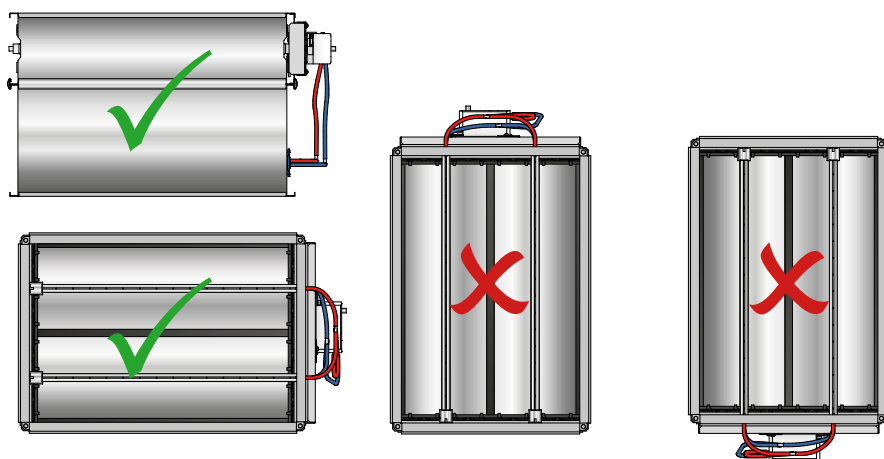
Figur 8. Montage - For rektangulære kanaler monteres spjældet altid således at regulatoren/aktuatoren er placeret langs med siden af kanalen.
