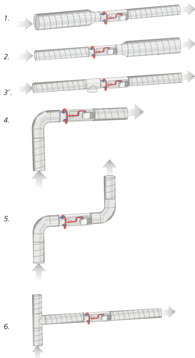
Figur 4. Krav til lige strækning i cirkulære kanaler, antal \emptyset inden produkt:
