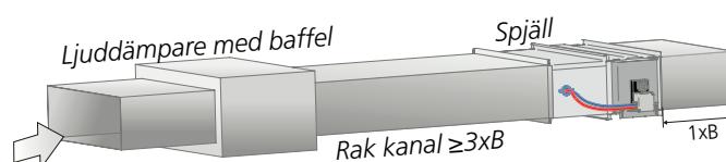
Figur 8. Krav på raksträcka 3 \times B vid ljuddämpare med baffel. Gäller både till- och frånluft.
