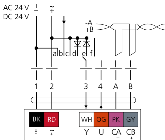
Figur 9. Kopplingsschema.
