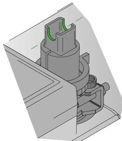
Figur 13. Urklipp i spjällaxel indikerar spjällets position.
