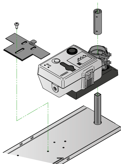
Figur 12. Demontering av spjällmotor.
