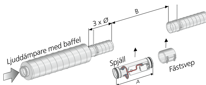
Figur 3. Krav på raksträcka 3 x \emptyset vid ljuddämpare med baffel eller centrumkropp.
