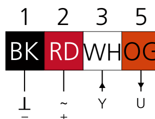
Kuva 2. KytKentä.
