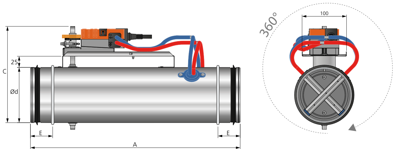
Kuva 3. Mitat (mm), REACT V BMP pyöreä. Pellit voidaan asentaa haluttuunkallistuskulmaan.
